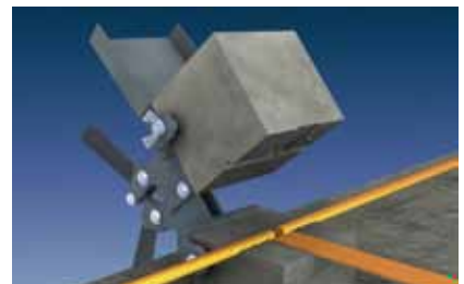
Soldadura aluminotérmica.
